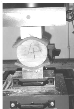
Abbildung 2: Mauerwerks-Prüfeinrichtung (IEMB)
