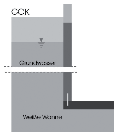
Abbildung 3: Weiße Wanne
