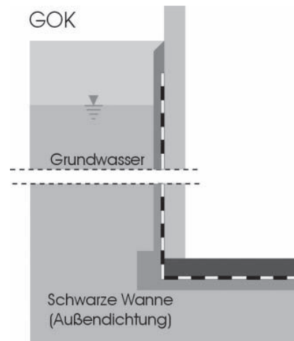
Abbildung 2: Schwarze Wanne
