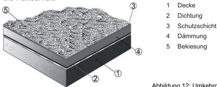
Abbildung 12: Umkehrdach
