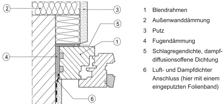
Abbildung 15: Detail zum dichten Anschluss des Blendrahmens an die Außenwand
