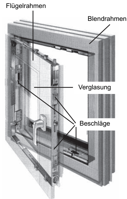
Abbildung 14: Hauptbestandteile eines Fensters
