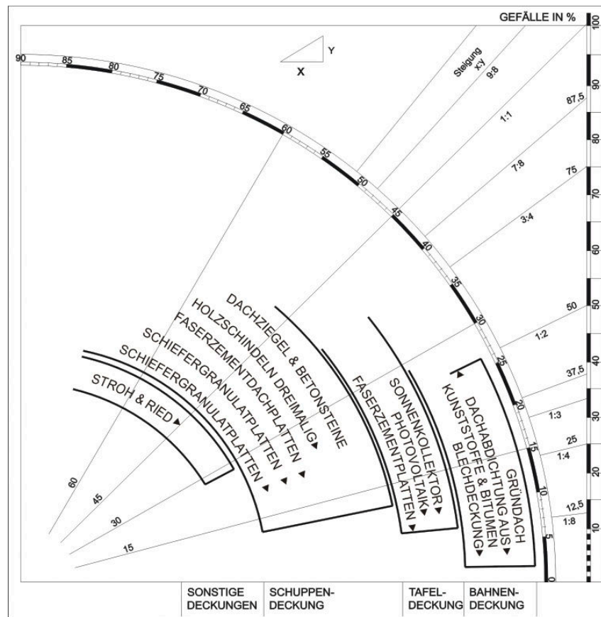
Abbildung 7: Grundtypen von Dachabdichtungsarten
