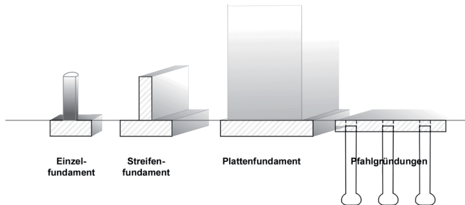
Abbildung 1: Fundamentarten
