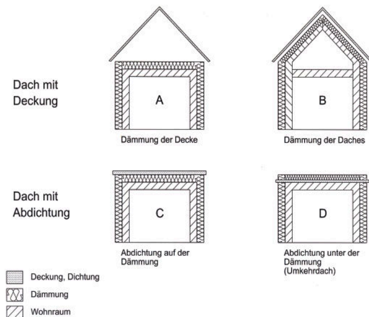
Abbildung 6: Grundtypen von Dachabdichtungsarten
