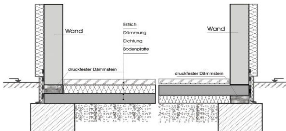
Abbildung 4: Dämmung oberhalb oder unterhalb der Bodenplatte
