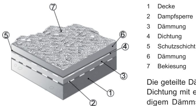
Abbildung 13: Kombinationsdach
