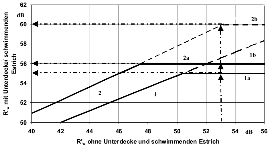
Bild 7: Verbesserung der Luftschalldämmung durch schwimmenden Estrich und/oder biegeweiche Unterdecke (Pfeilmarkierungen siehe nachfolgendes Beispiel)
