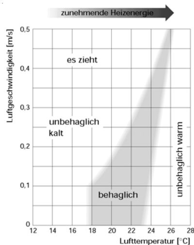
Bild 1: Behaglichkeitsdiagramm [1]
